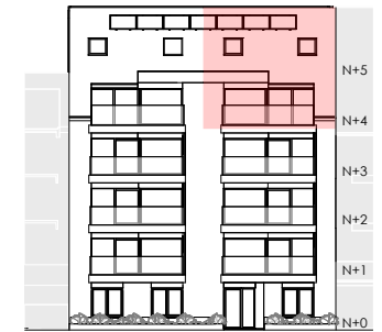
VOORGEVEL
