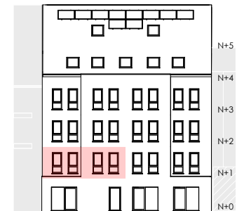
ACHTERGEVEL
