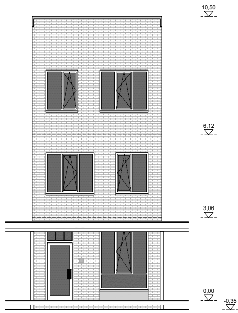
Voorgevel
