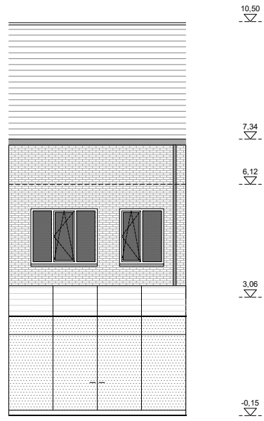
Achtergevel
