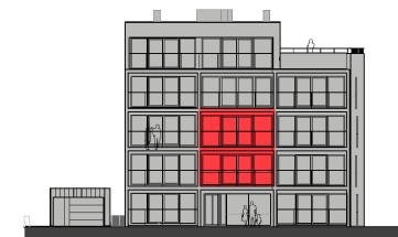
VOORGEVEL
